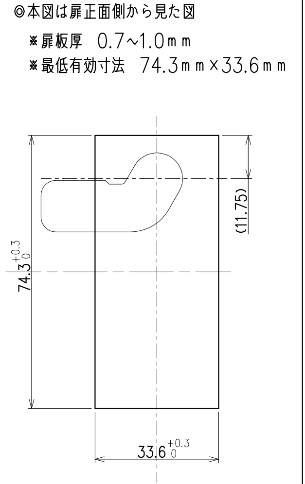
取付け穴寸法図
