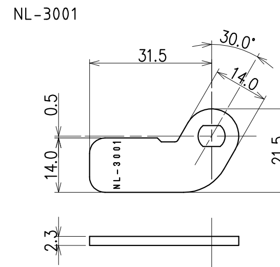
カンプレート詳細図
