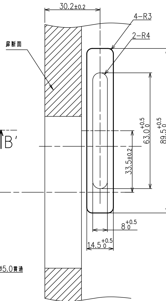
A-A' 断面図
