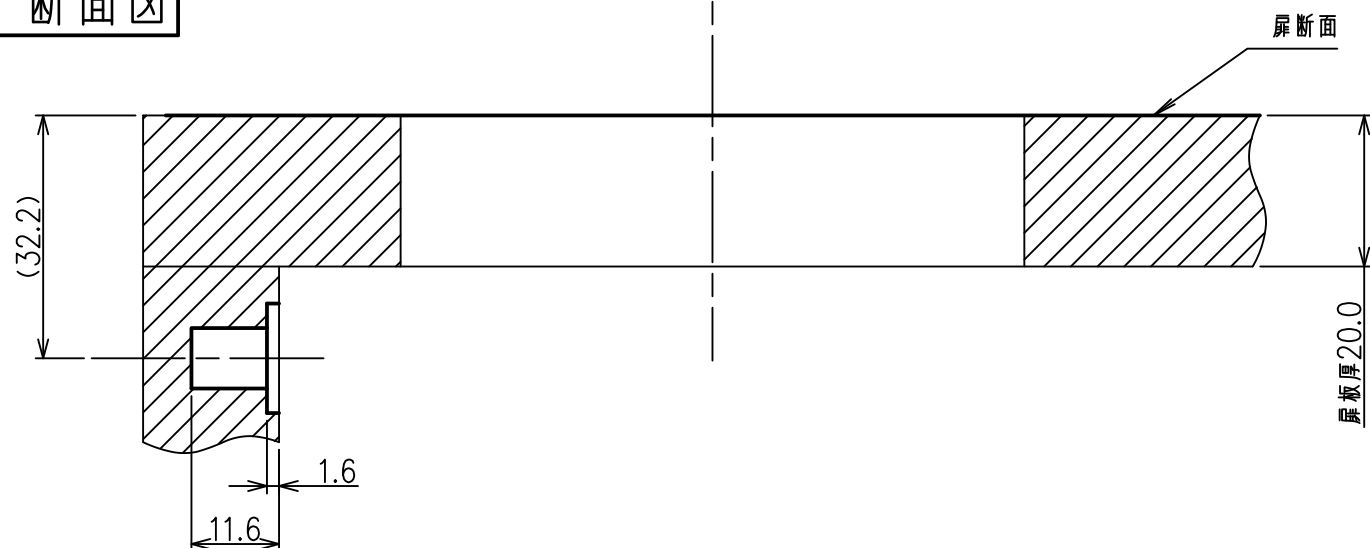
B-B' 断面図
