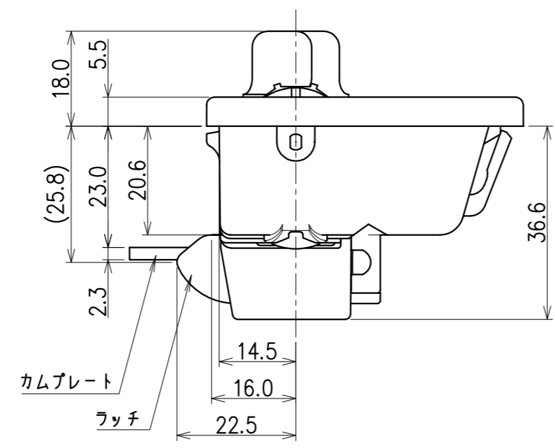
下面図
