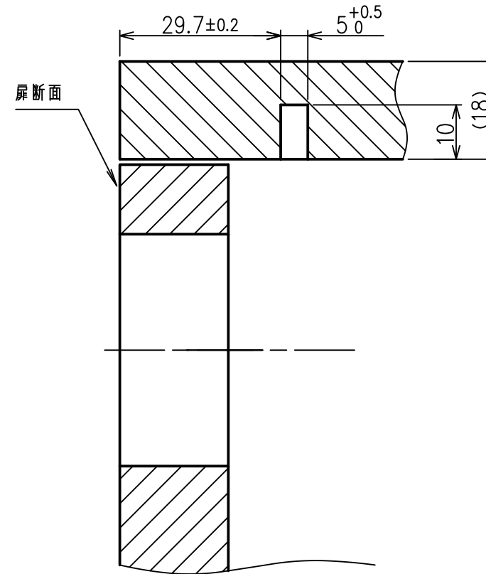
A-A 断面図
