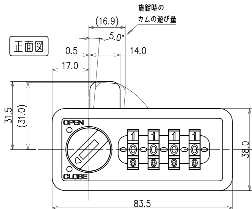
右側面図
