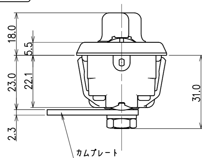
下面図
